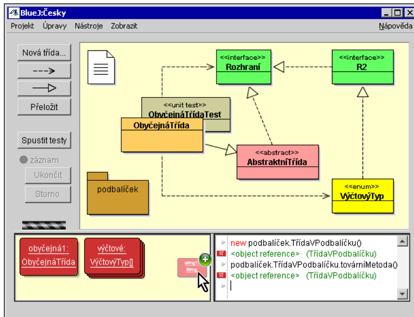
Obr. 12: Odkaz získaný v příkazovém panelu lze zkopírovat do zásobníku odkazů
