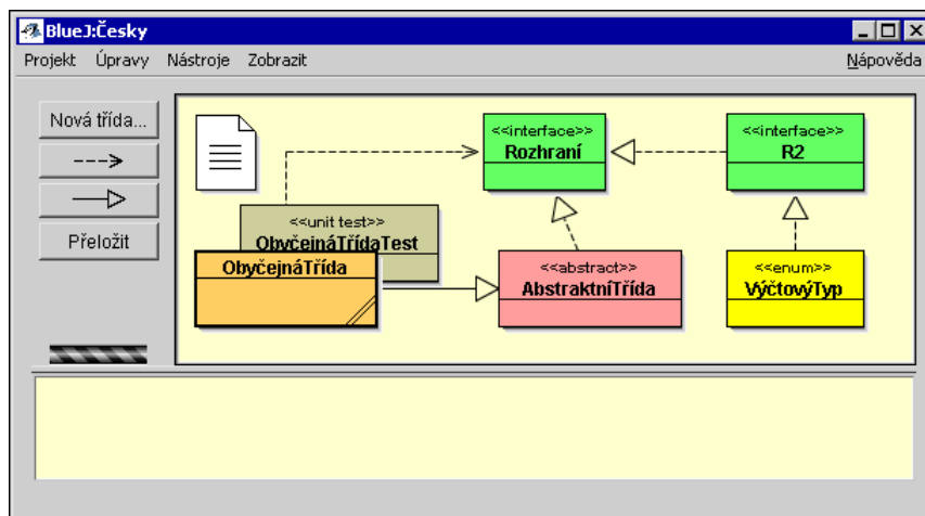
Obr. 1: Aplikační okno
