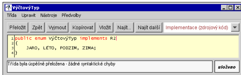
Obr. 2: Okno editoru
