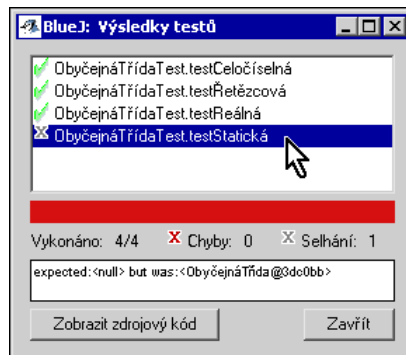
Obr. 11: Okno zobrazující výsledky provedených testů
