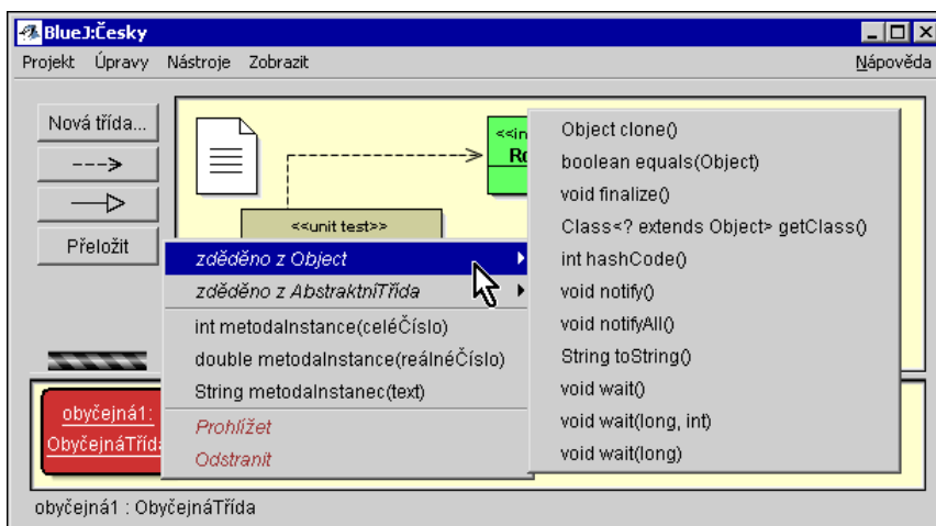
Obr. 5: Místní nabídka odkazu na instanci
