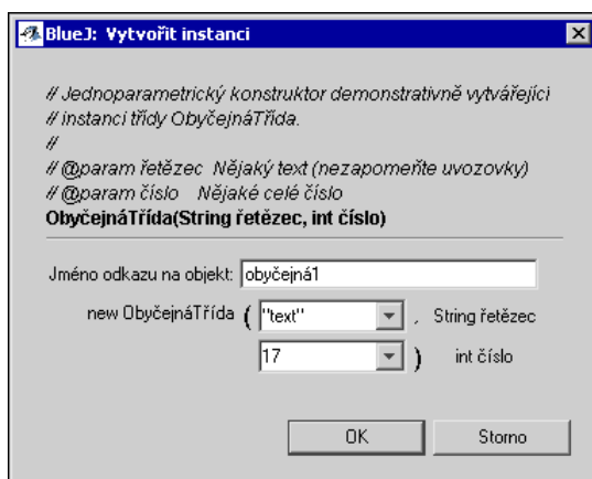
Obr. 4: Okno pro zadání hodnot parametrů konstruktoru
